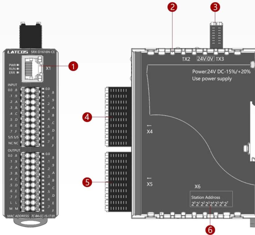
图 4 模块接线图
